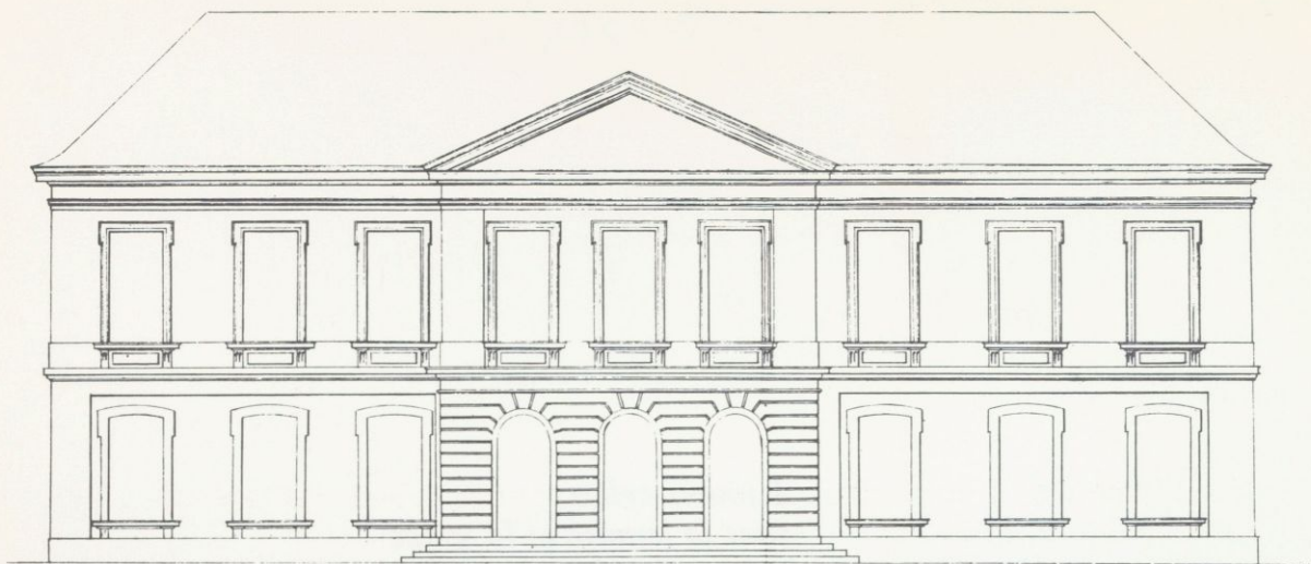
Hôtel de La Marck. Façade côté jardin. Dessin, 1760. Arch. nat. Minutier central LXXXIII, 467.
